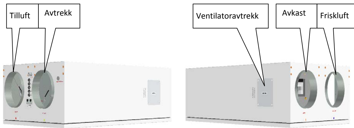
(Skisse viser AHU-400 HV1)
